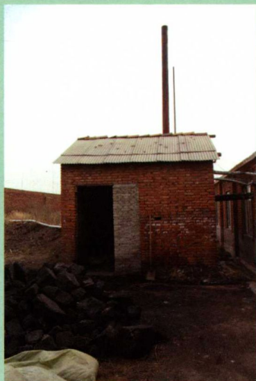
鸡舍供暖系统—锅炉房
