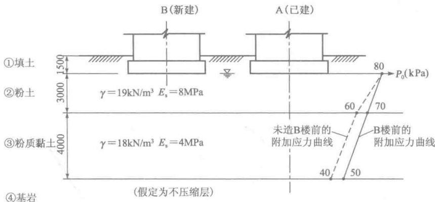
题 10 图(尺寸单位:mm)
