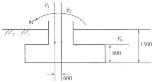
题 12 图(尺寸单位:mm)
