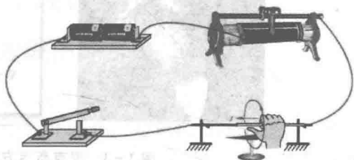
图 1-1 奥斯特实验
