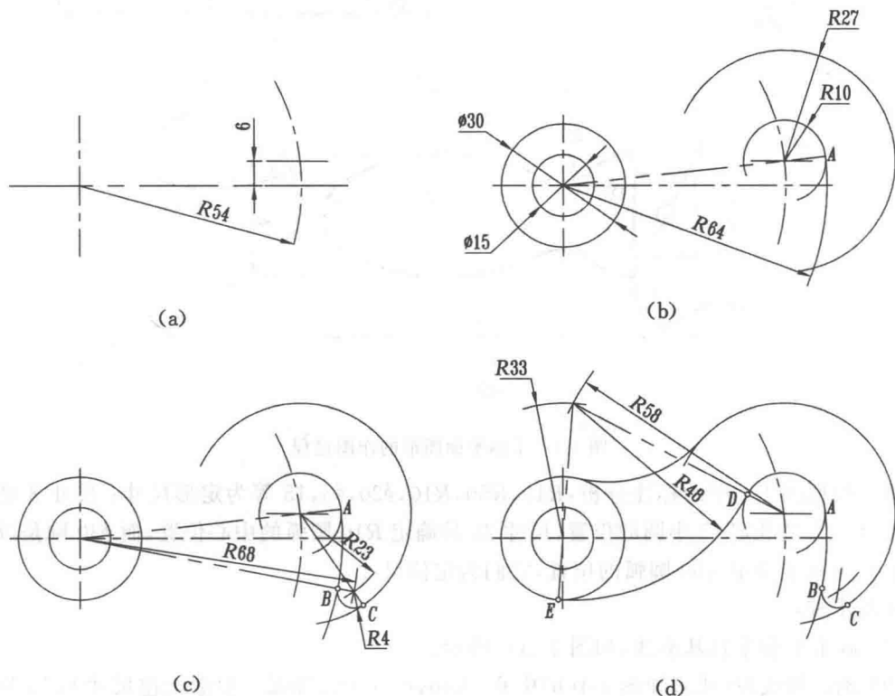
图 1-6 爪钩平面图形的作图过程
