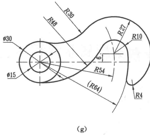
图 1-6 爪钩平面图形的作图过程(续)
