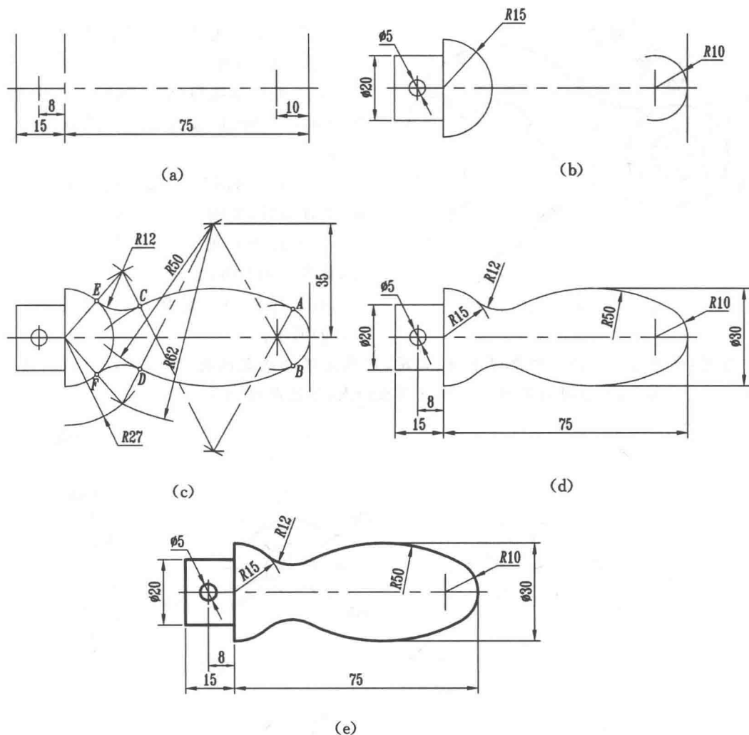
图 1-4 手柄平面图形的作图过程
