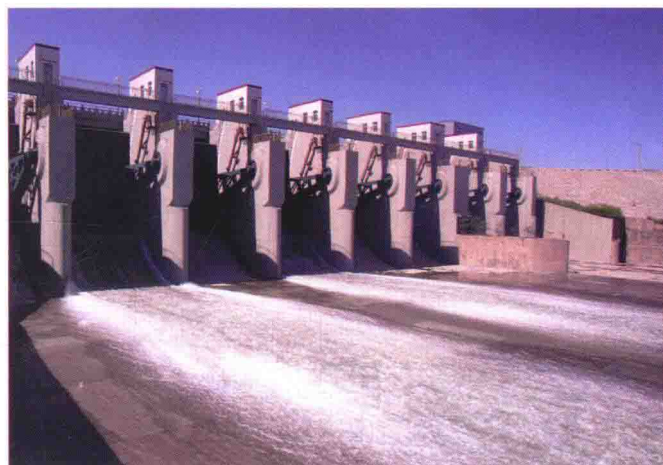
水库正常溢洪道
