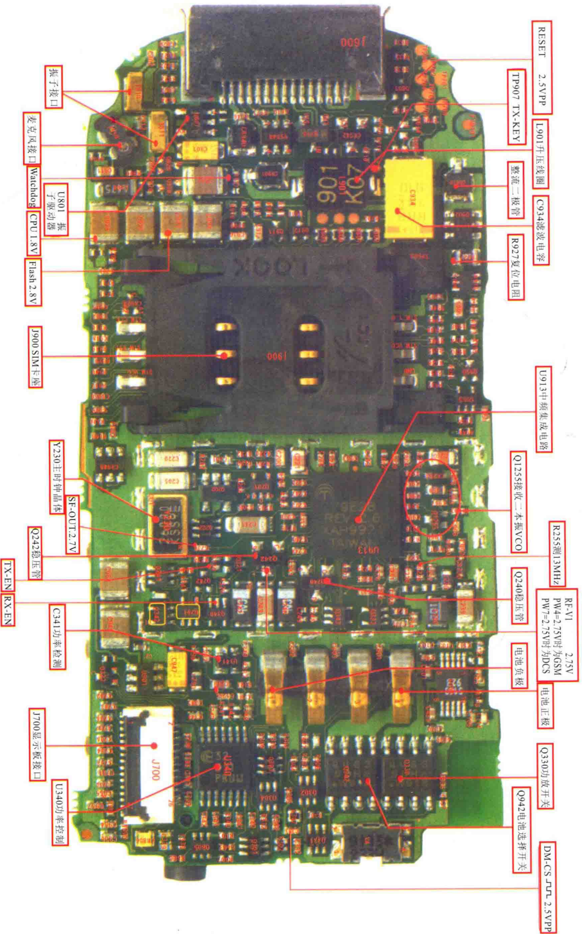
摩托罗拉V988手机元件实物图A面
