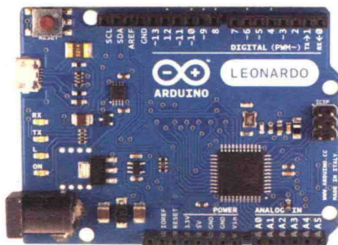
图 1.4 Arduino Leonardo
