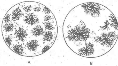
第一圖 金鯽魚鱗片之顯微鏡觀
