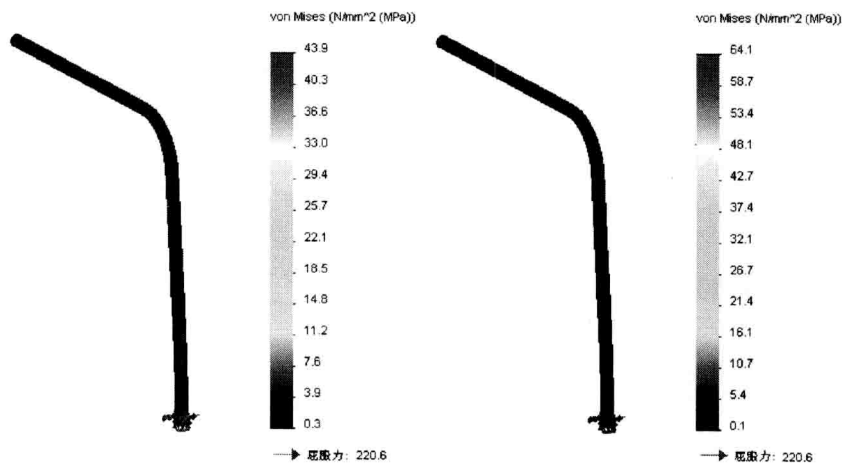
图 1-5 应力结果
