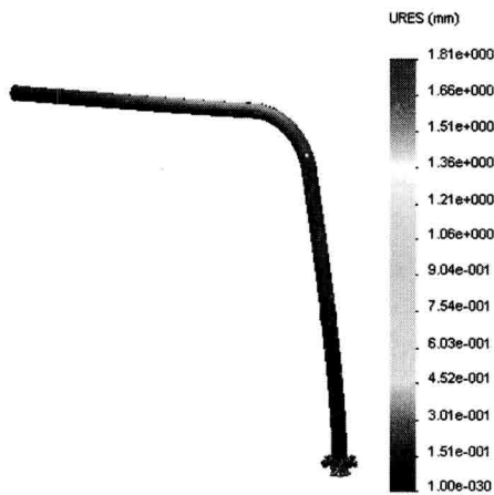
图 1-16 位移结果
