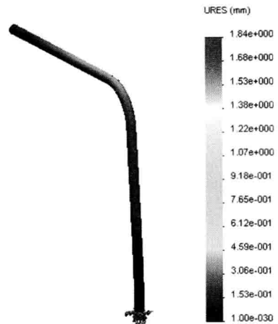
图 1-6 位移结果
