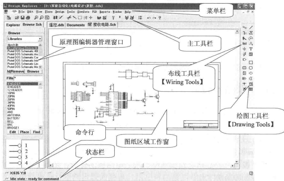
图 1-1 原理图编辑器
