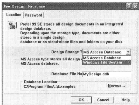
图 1-11 两种文件存储方式
