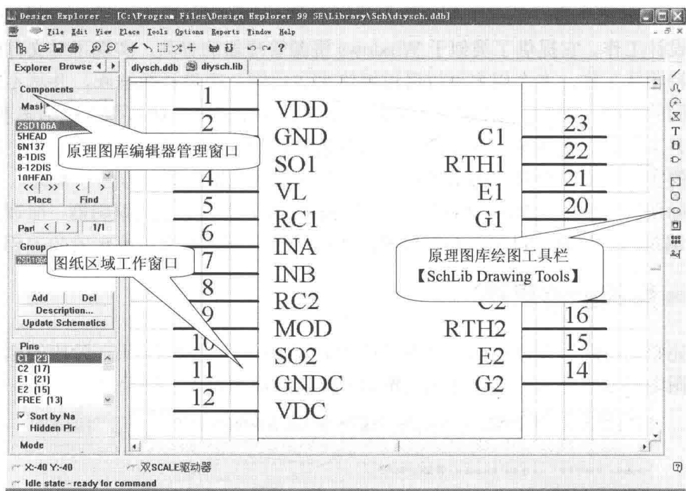
图 1-2 原理图库编辑器
