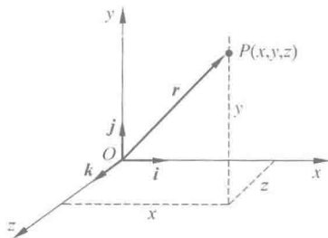
图 1-2 位置矢量
