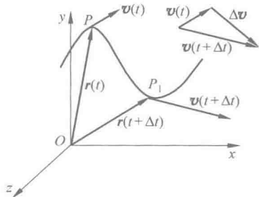
图 1-5 平均加速度矢量
