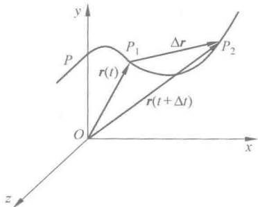
图 1-3 位移矢量
