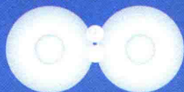
氢分子
