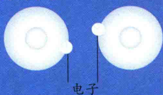
2个氢原子
