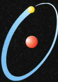
卢瑟福的原子模型
