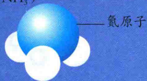
氨分子 (NH 3 )
