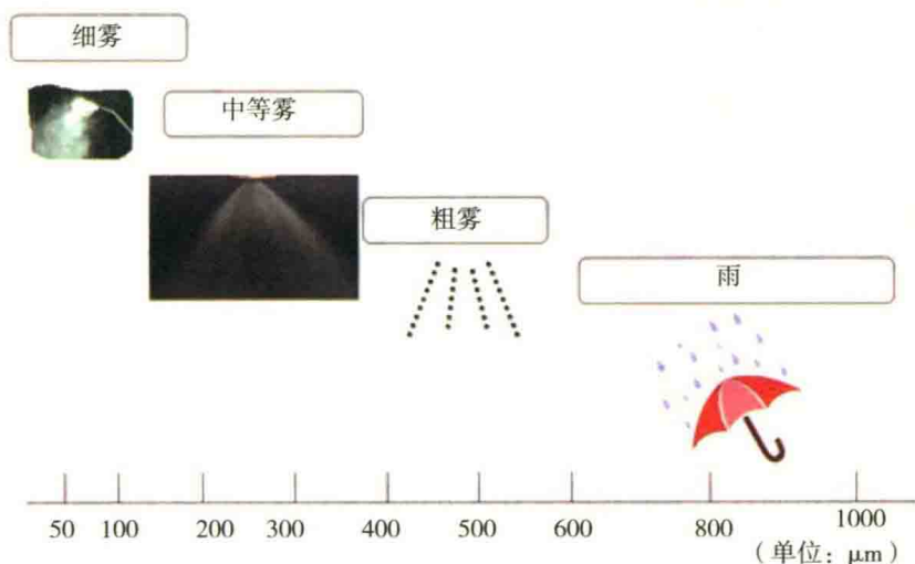
图 1-2 不同喷雾方式所对应的雾滴粒径
