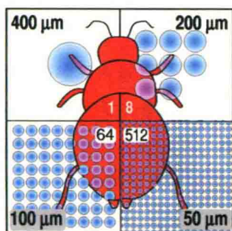
图 1-4 雾滴粒径与雾滴数的关系
