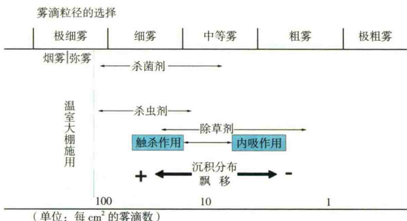
图 1-6 不同类型农药所应采用的喷雾方式
