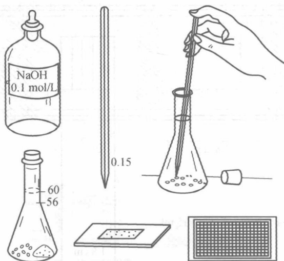
图 1-4 斯陶尔氏法示意(单位: mL)
