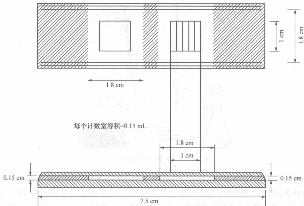
图 1-3 麦马斯特氏计数板示意
