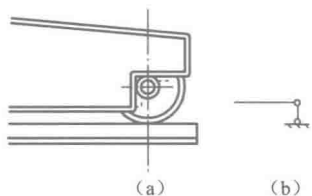
图 2-1 活动铰支座
