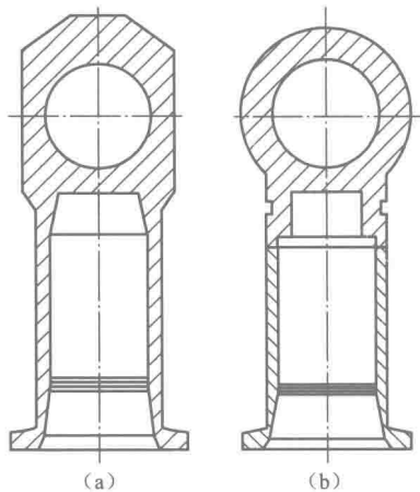
图 1-4 锻件改为铸锻焊结构 (a) 较差结构; (b) 改进结构
