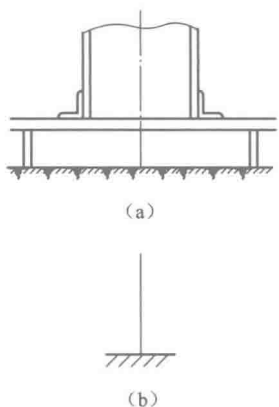
图 2-3 固定支座
