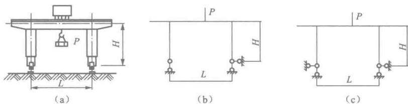
图 2-5 龙门起重机
