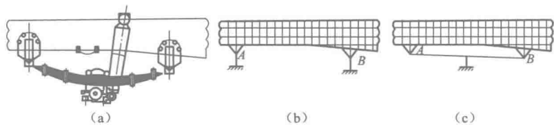
图 2-6 车架
