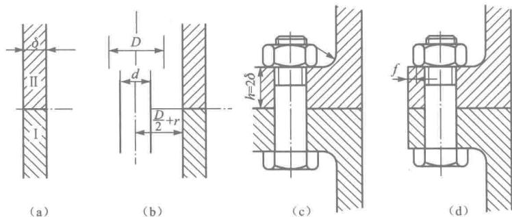
图 1-10 螺栓连接结构设计
