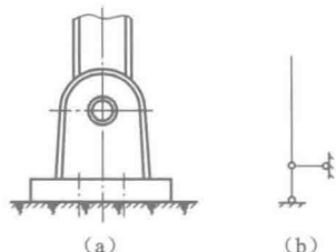
图 2-2 固定铰支座
