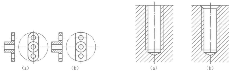
图 1-7 凸缘结构
