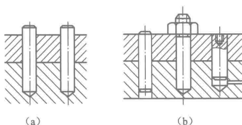
图 1-1 保证销钉容易装拆 (a) 错误结构; (b) 改进结构
