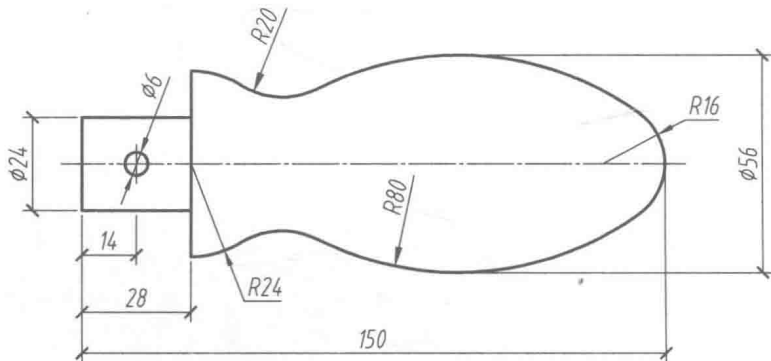
图 10101 手柄平面图
