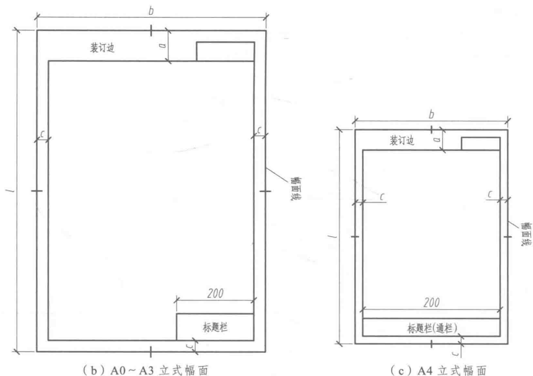
图 10110 图框格式
