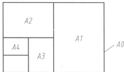
图 10109 各种图纸图幅的尺寸关系
