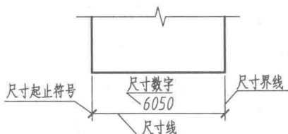
图 10117 尺寸标注的组成
