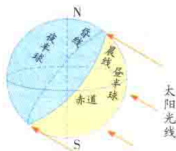
晨昏线示意
