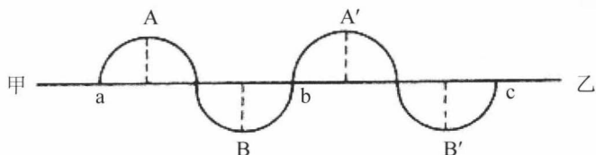
图 1.2 音波示意图
