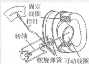
(c) 电动式仪表测量机构
