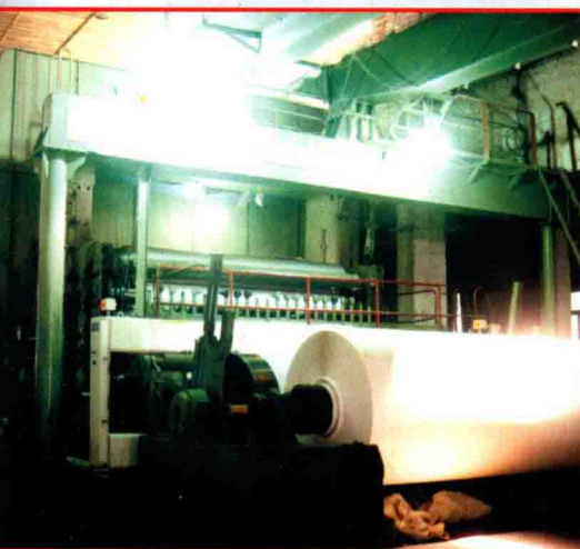
胶印书刊纸生产线
