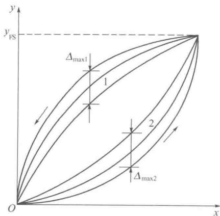
图 1-6 传感器重复性示意图
