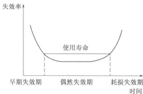
图 1-7 故障率变化曲线
