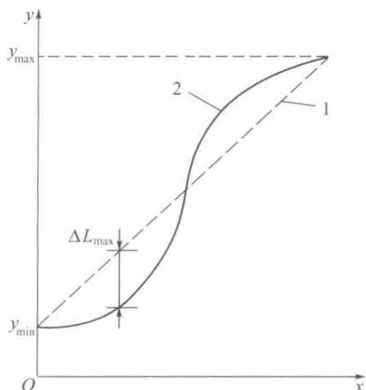
图 1-4 传感器线性度示意图
