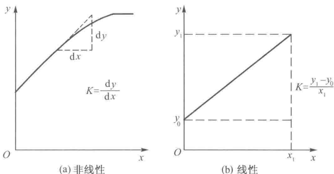
图 1-3 传感器灵敏度示意
