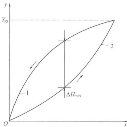
图 1-5 传感器迟滞特性示意图
