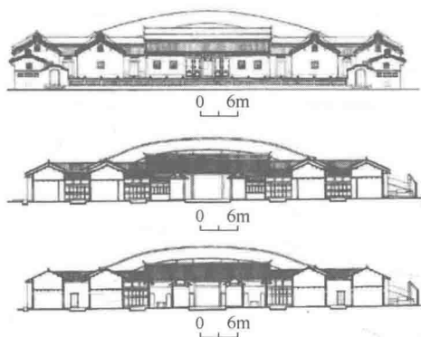
图 1-5 客家围龙屋
