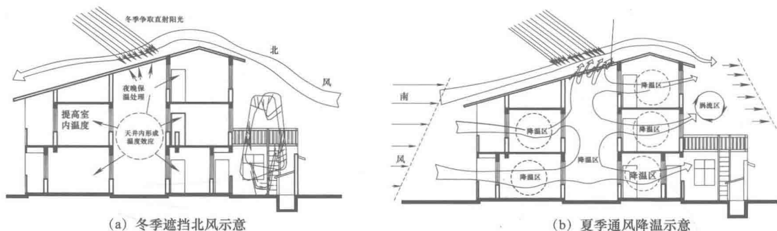
图 1-8 带有可开启活动玻璃屋顶的天井内庭
