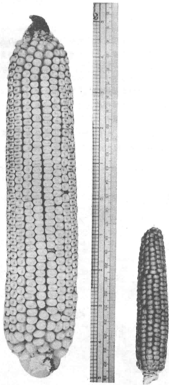
图2 大约1500年前在科罗拉多州卡顿伍德（Cottonwood）种植的竹篮人（Basketmaker）玉米穗与现代改良的马齿种玉米穗的对照。竹篮人玉米穗长约43~44英寸，现代玉米穗长约97~98英寸，竹篮人玉米穗的长度还不到现代玉米的平均长度。
