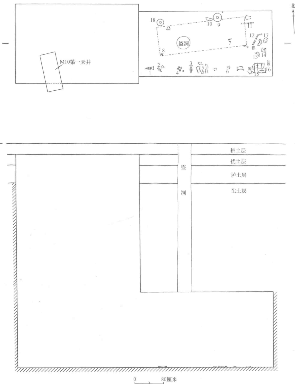
图二 M9墓葬平、剖面图
