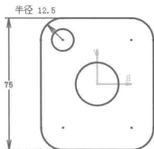
图 4.8 添加竖直约束
