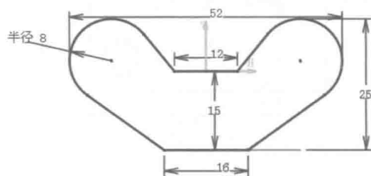
图 3.8 添加半径约束
