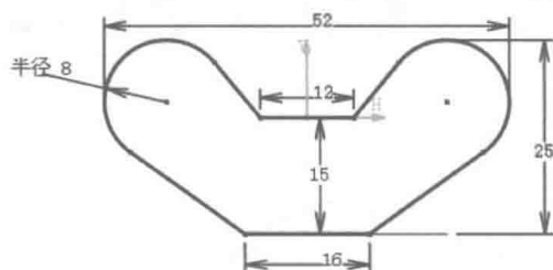
图 3.1 草图 3
