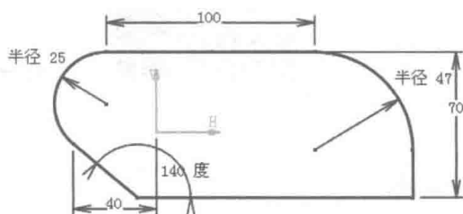
图 1.6 标注竖直尺寸
