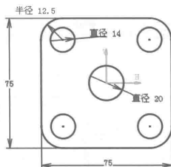
图 4.1 草图 4
