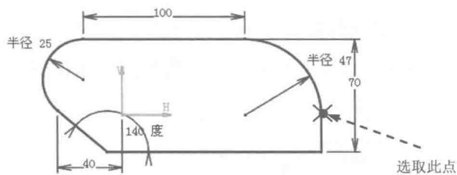
图 1.7 约束相合
