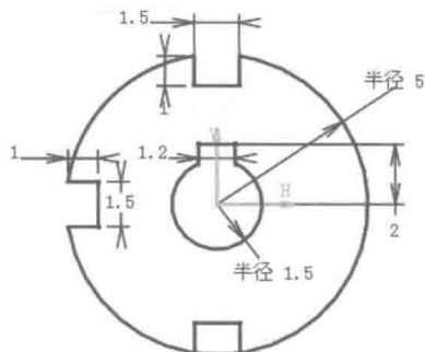
图 2.7 镜像
