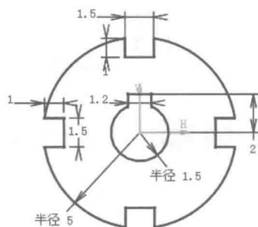
图 2.1 草图 2
