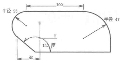
图 1.5 标注水平尺寸
