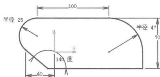
图 1.1 草图 1
