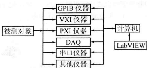
图 1-7 虚拟仪器系统的典型组成
