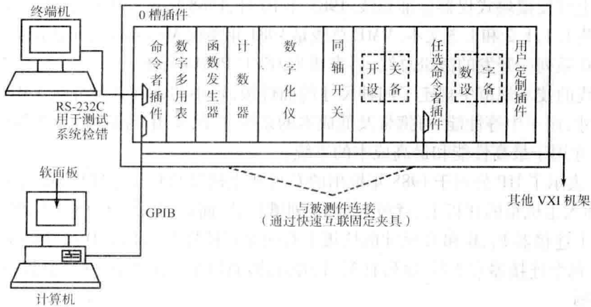
图1-4 VXI 仪器系统实例
