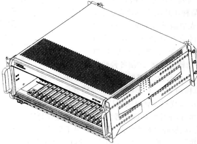
图 1 - 5 18 槽 PXI 机箱
