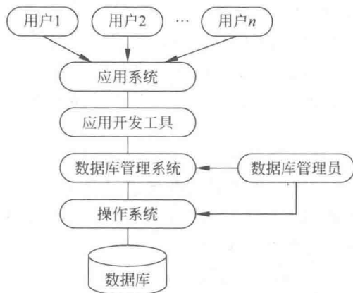
图 1.1 数据库系统
