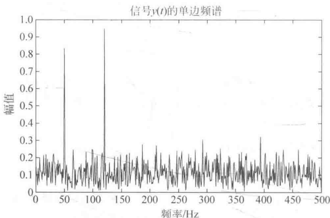
图 2.9 受干扰信号的单边频谱图
