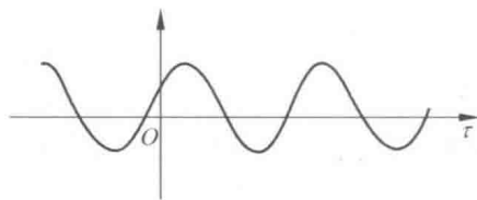
图 2.6 同频正弦信号的相关函数波形
