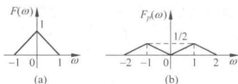
图 2.5 f(t) 与 f_p(t) 频谱图
