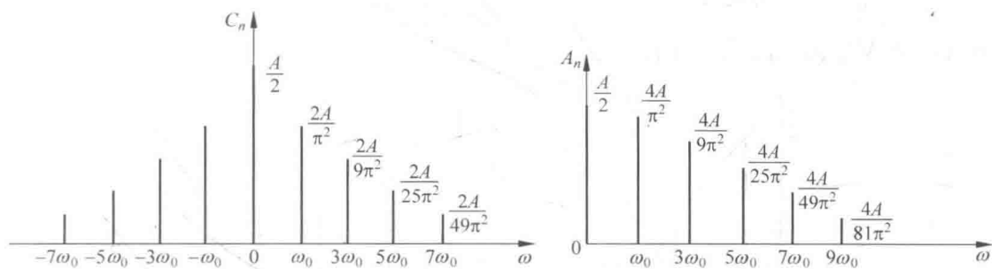
图 2.2 三角脉冲信号 x(t) 的幅值谱
