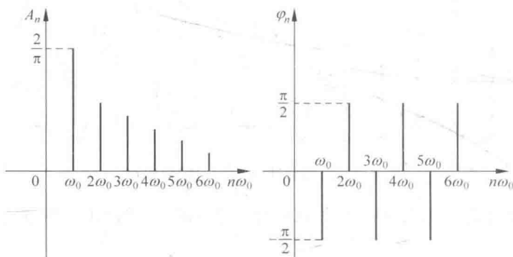
图 2.4 x(t) 的频谱与相谱
