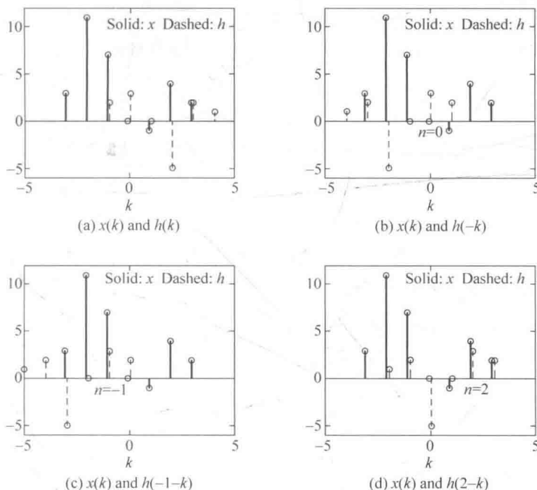
图 2.10 离散信号卷积过程图
