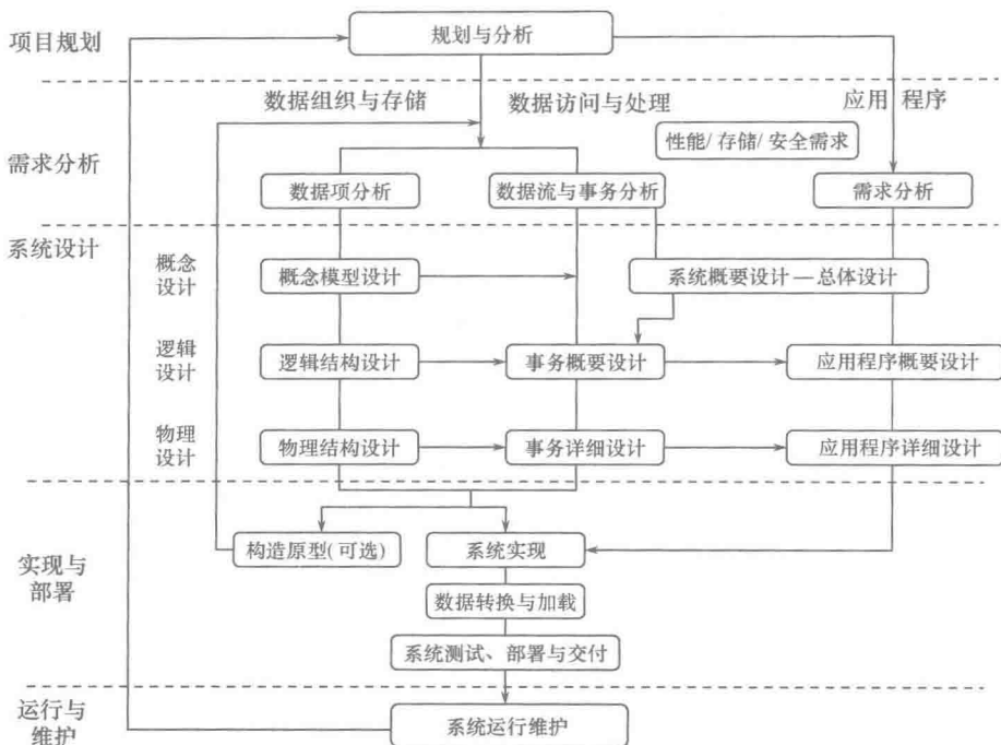
图 1.1 数据库应用系统生命周期模型
