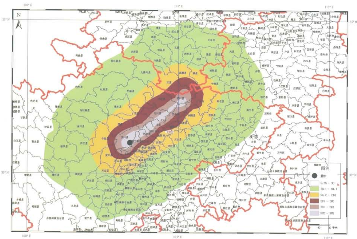
汶川8.0级特大地震主震PGA(东西向)分布图 (来源于四川防震减灾信息网)
