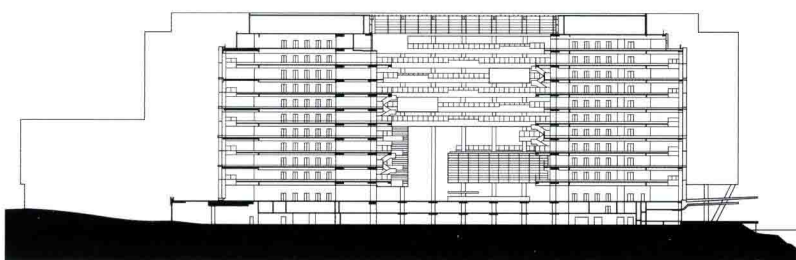
Section 剖面图
