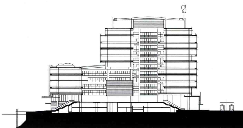
Section 剖面图
