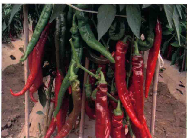
彩图46 ( 辣 椒 )
