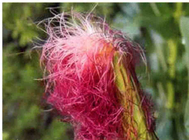
彩图103 ( 玉米须 )
