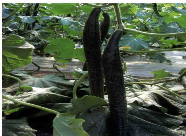
彩图29 (黄瓜)
