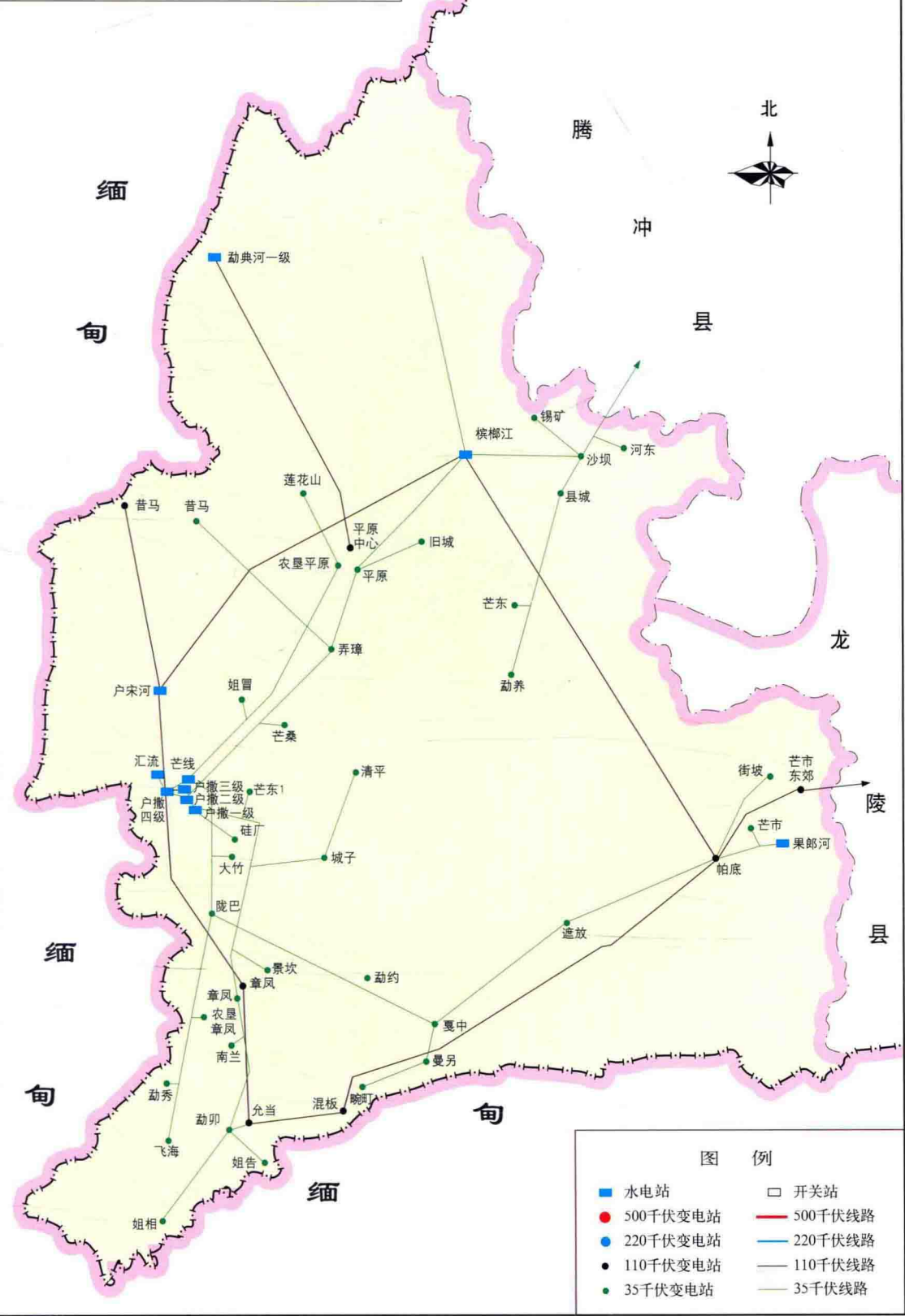
德宏电力系统接线示意图 (1998年)
