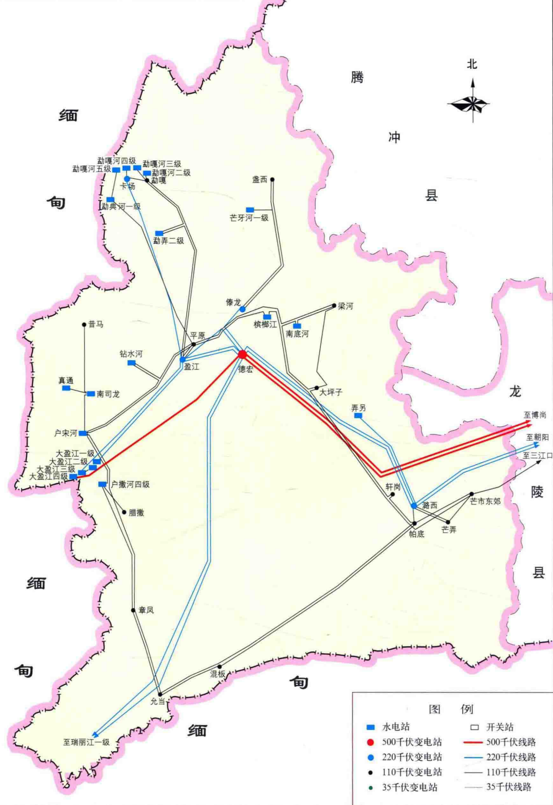
德宏电力系统接线示意图（2008年）
