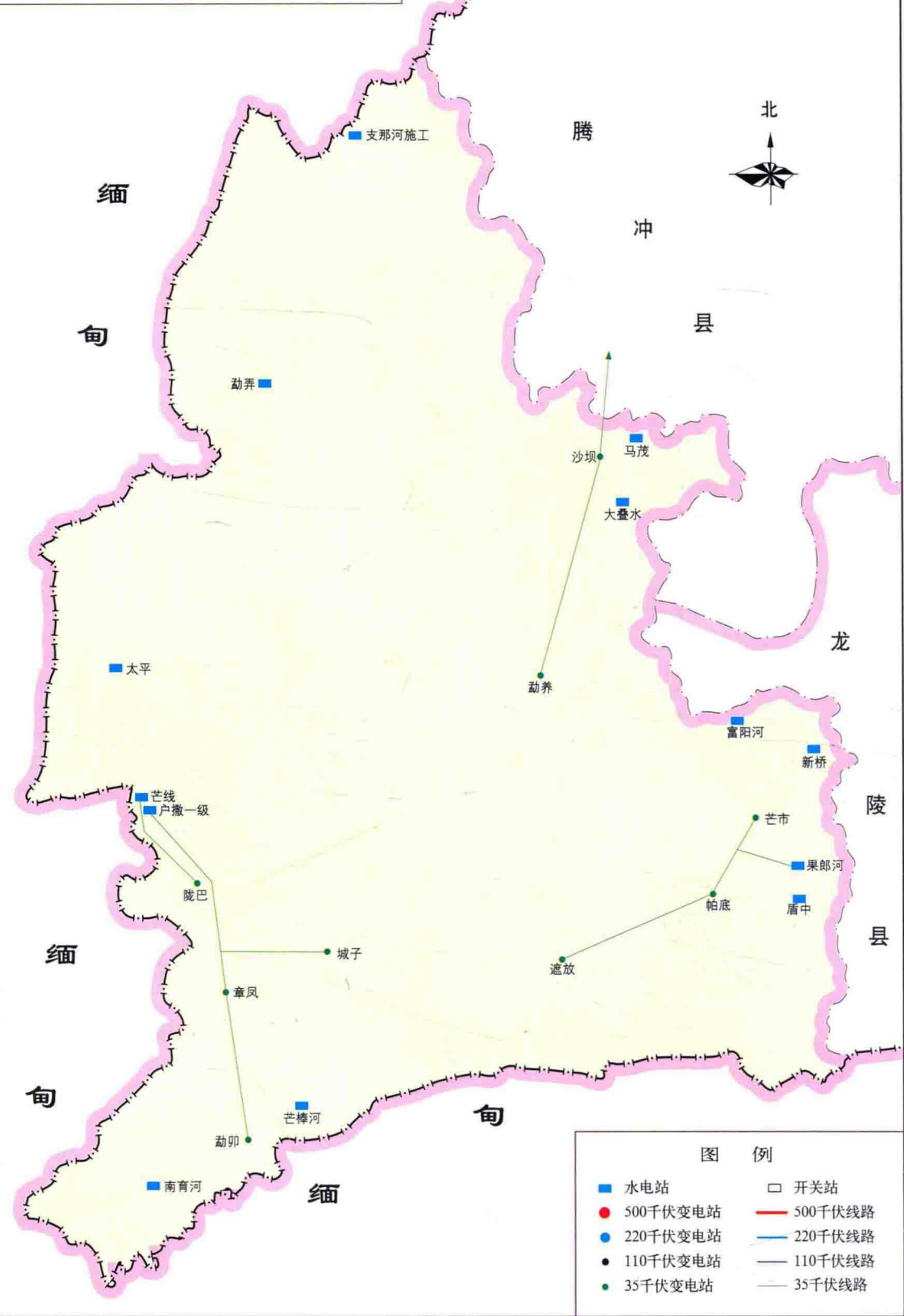
德宏电力系统接线示意图 (1984年)
