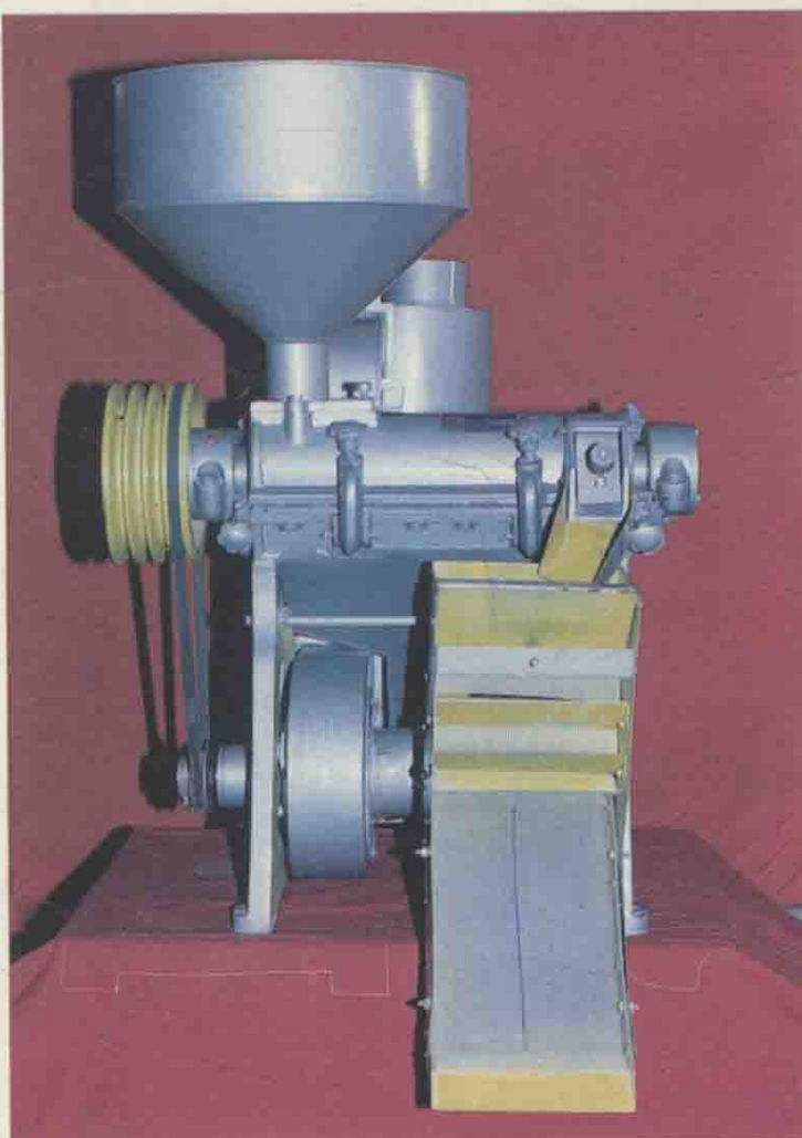
6NF-9.5 型碾米机
