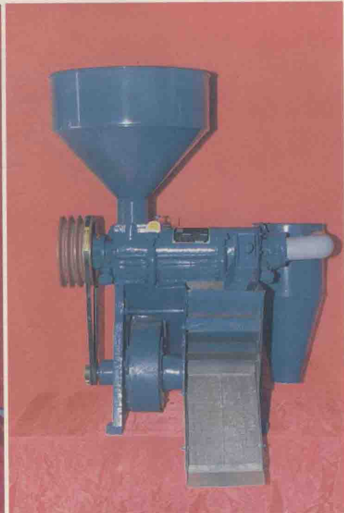
6NPF-9.5 型喷风碾米机
