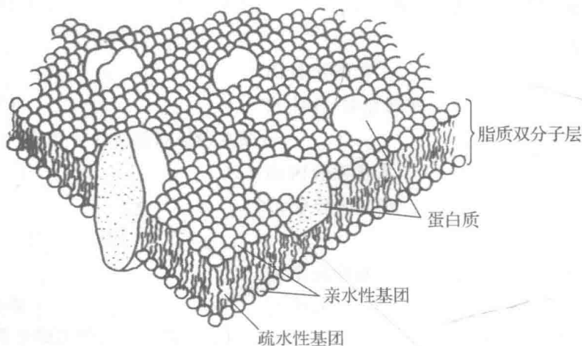
图 2-1 膜的液态镶嵌模型
