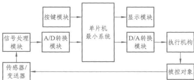
图 1-2 典型的单片机控制系统方框图
