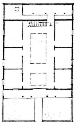
首层平面
