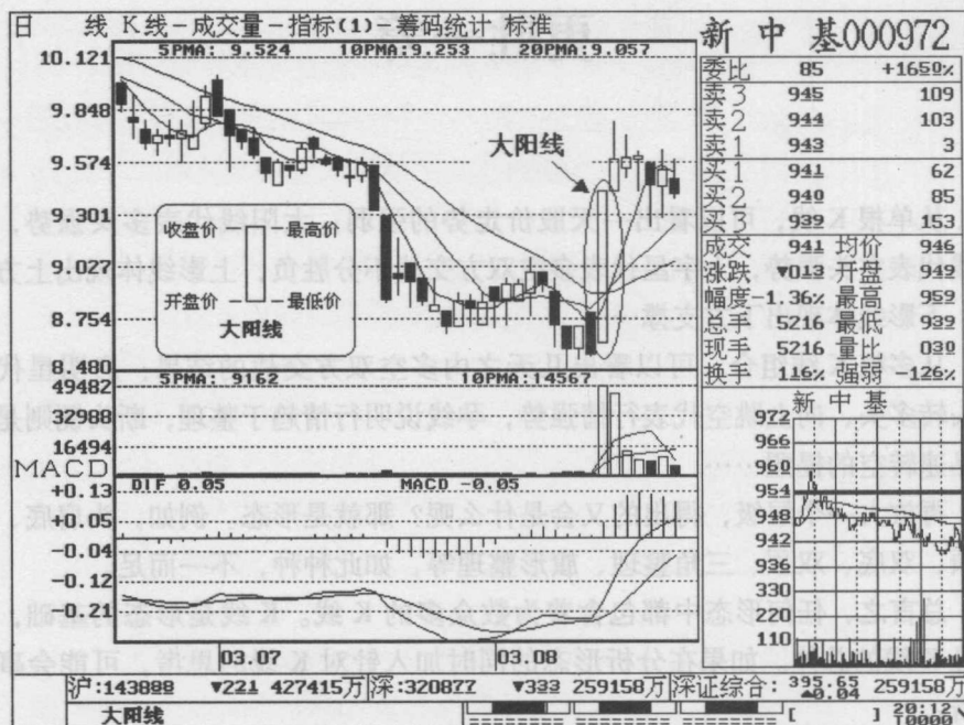
图 1-1 大阳线
