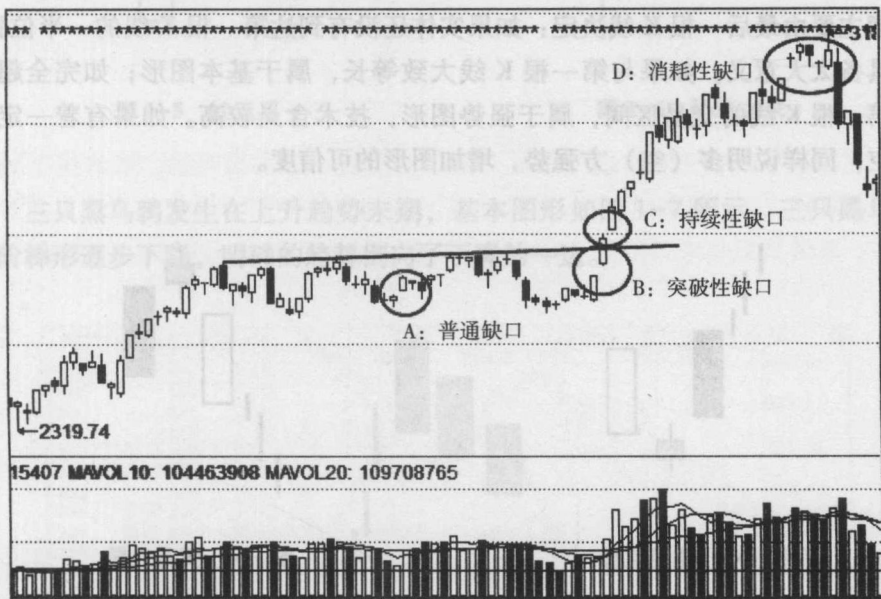
图 1-2 四种缺口
