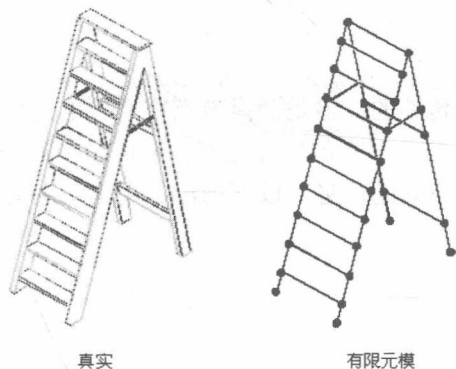
图 1-1 有限元模型
