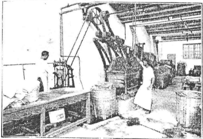
(6) 壓堅機 用蒸汽壓堅，即成粗胚。
