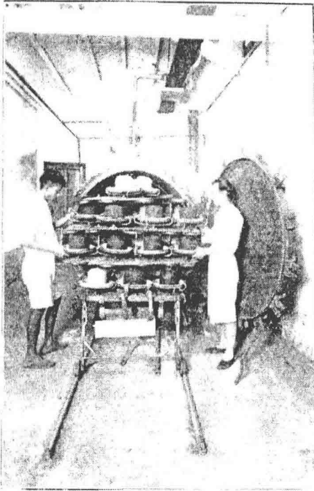
(11) 烘帽機 經烘帽爐烘 過之呢帽， 雖雨濕不變 式樣，此為 特色。普通 小規模製帽 廠，並無此 種設備。
