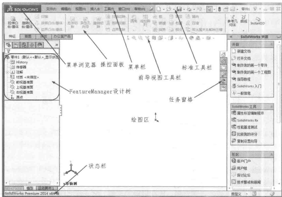
图 1-2 SolidWorks 2014 界面
