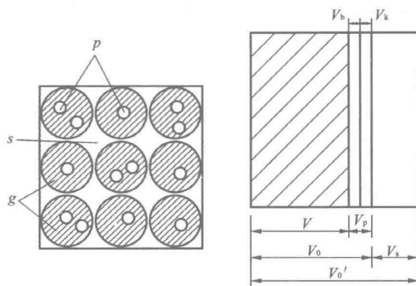
图 2.2 散粒材料堆积状态体积组成示意图
