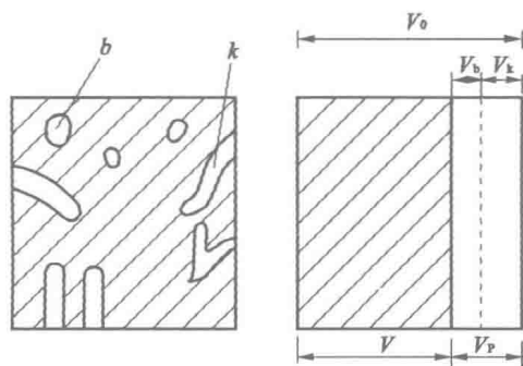
图 2.1 含孔材料体积组成示意图
