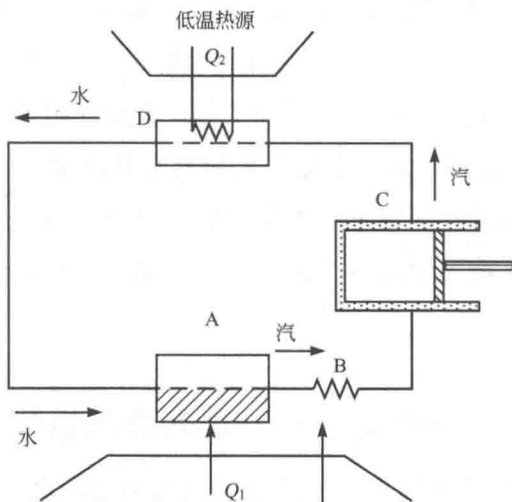
图 1.2 蒸汽机工作原理图
