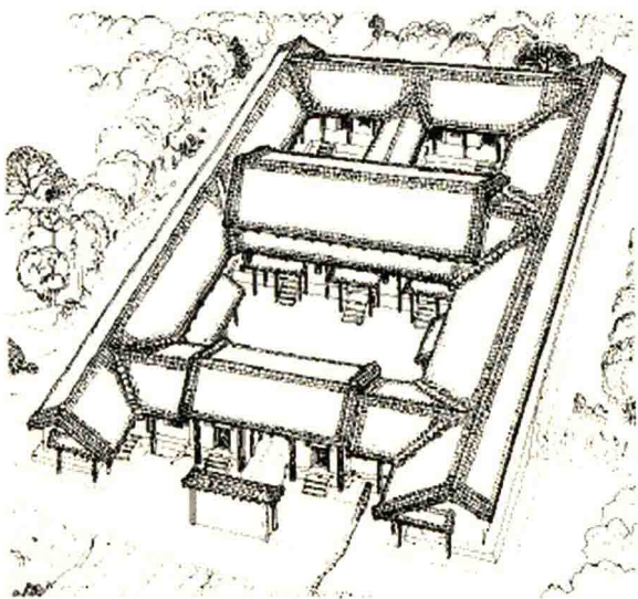
图 1-1-7 周原四合院建筑遗址复原图（傅熹年 提供）
