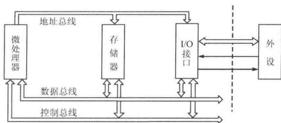
图 1-8 微型计算机结构
