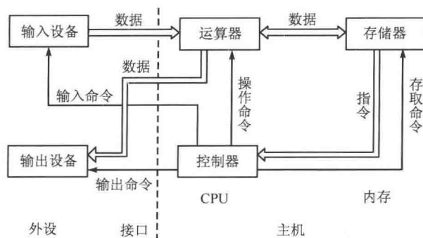
图 1-7 微型计算机硬件结构框图
