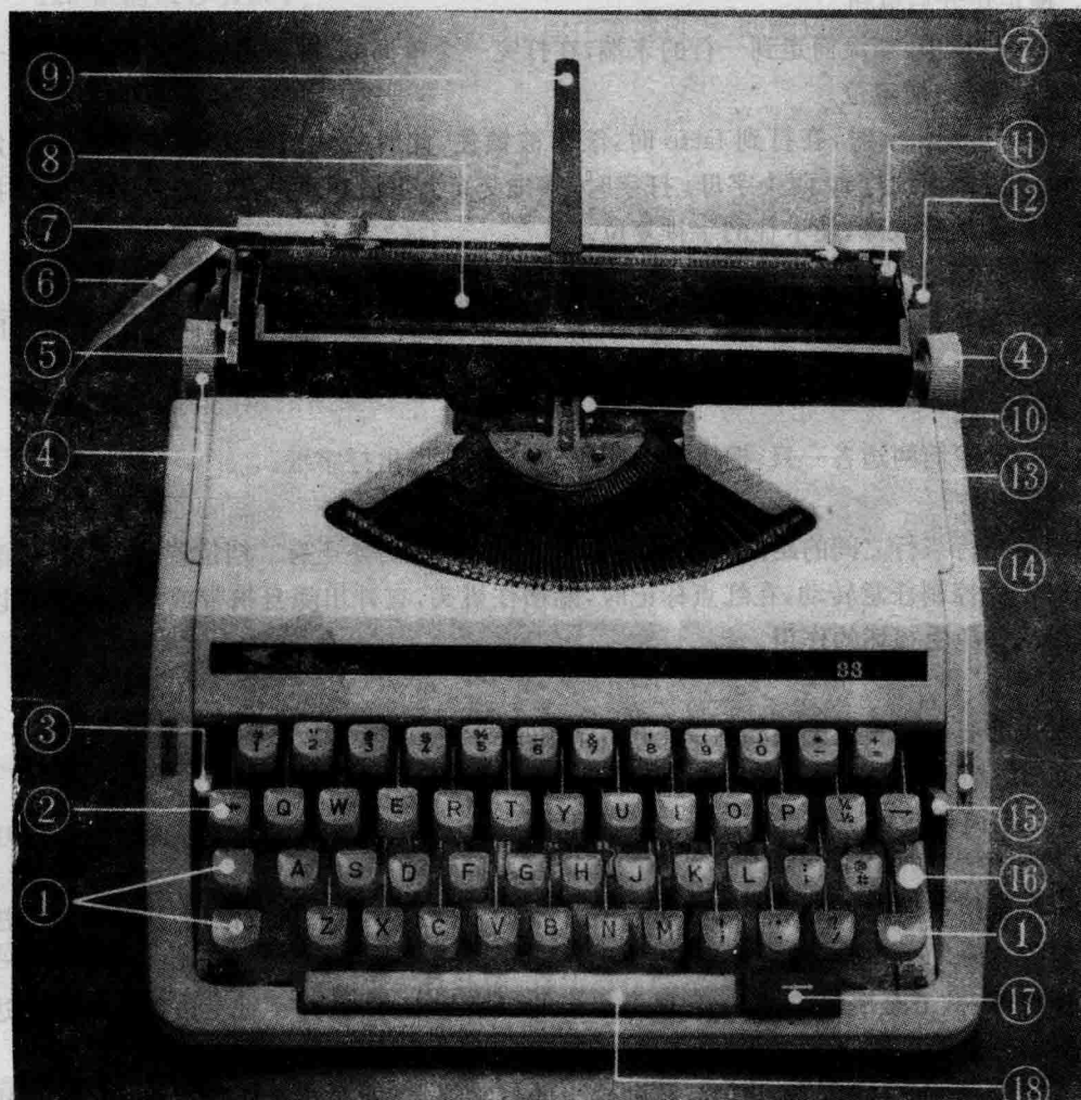
图1 打字机件名称
