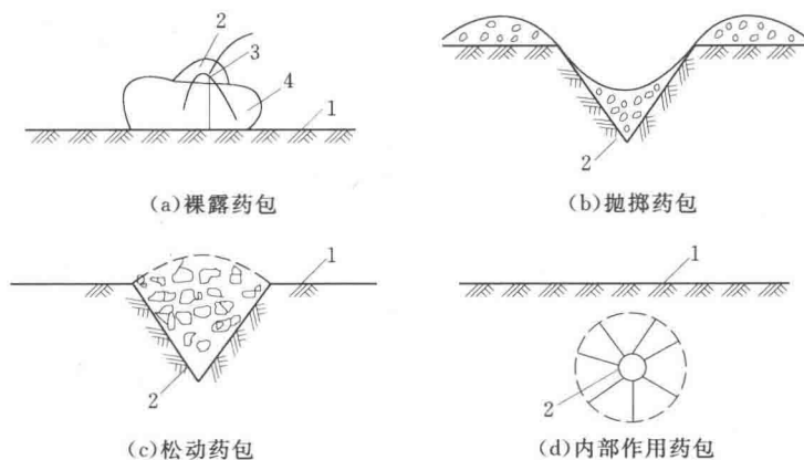
图 1.3 爆破作用分类
