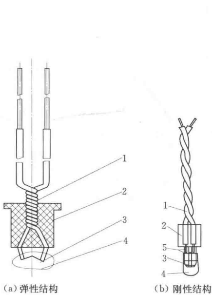
图 1.6 电引火元件结构示意图
