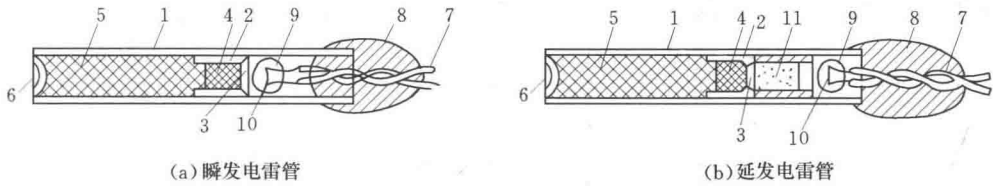
图 1.5 电雷管结构图
