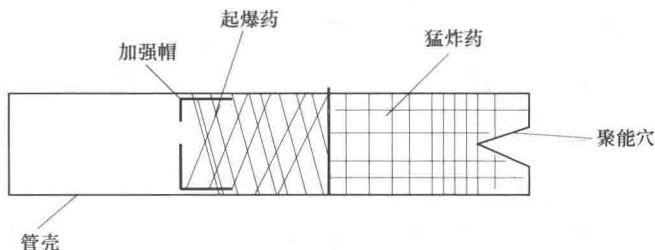
图 1.4 火雷管结构图
