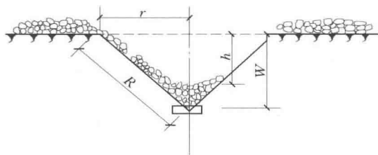
图 1.2 爆破漏斗
