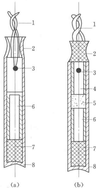
图 1.7 普通延期电雷管结构
