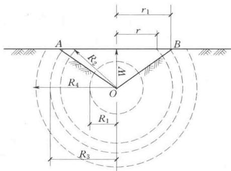
图 1.1 爆破影响范围示意图
