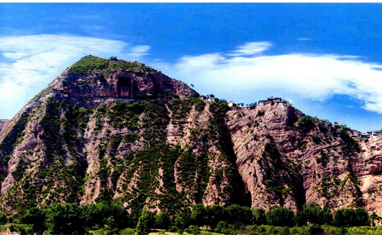
大像山石窟
