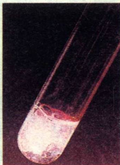
图 8-9 锌与盐酸的反应
