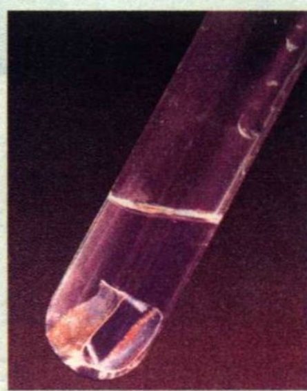
图 8-11 铜放入盐酸中
