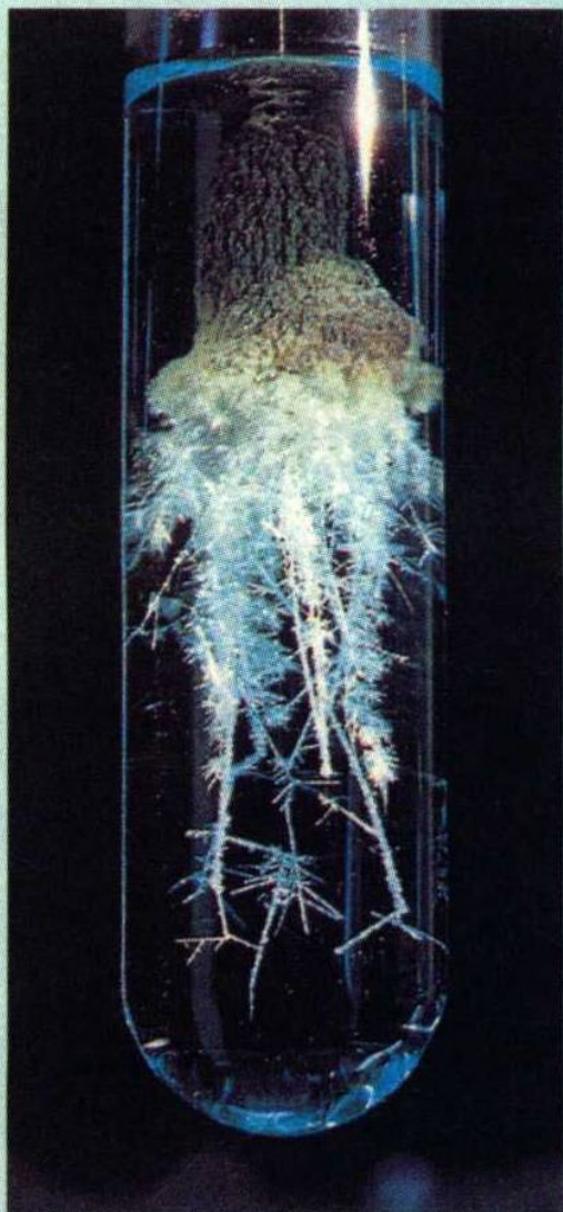
图 8-14 铜与硝酸银溶液的反应
