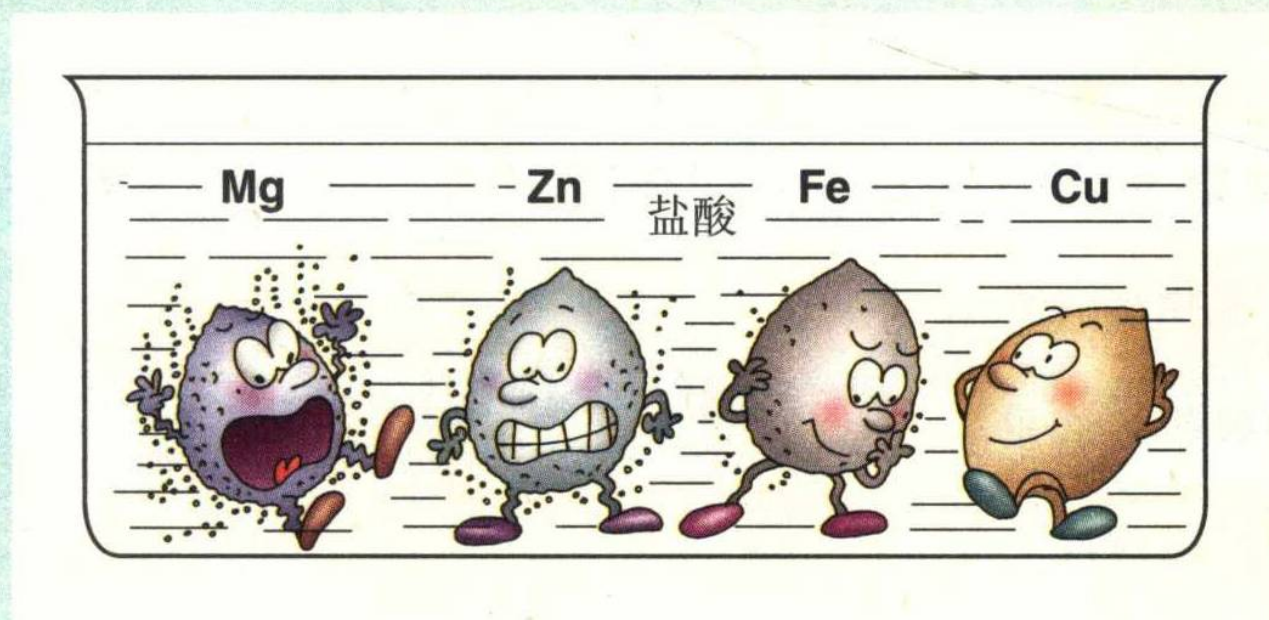
图 8-12 金属与盐酸反应的比较
