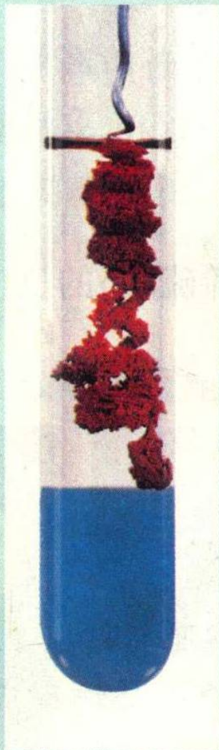
图 8-13 铝与硫酸铜溶液的反应
