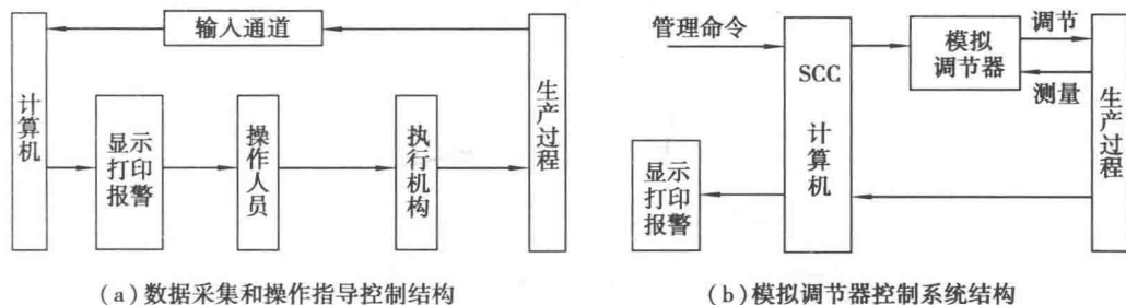
图 1.1 SCC 系统结构
